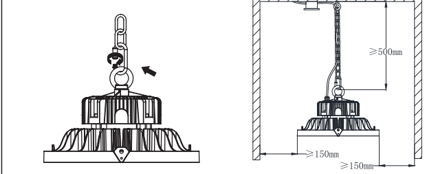
2- Pendant Mount
