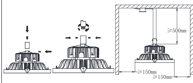
2- Pendant Mount
